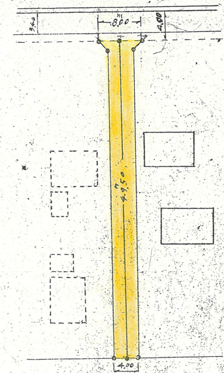
測量図
