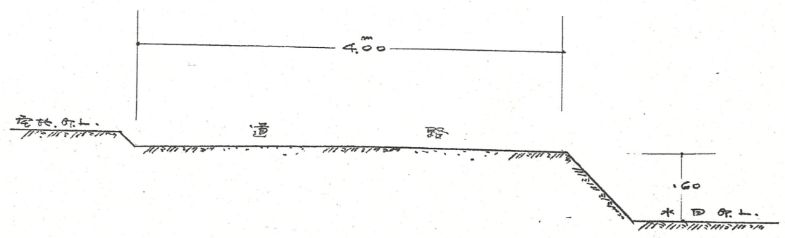
実測平面図 1/300
