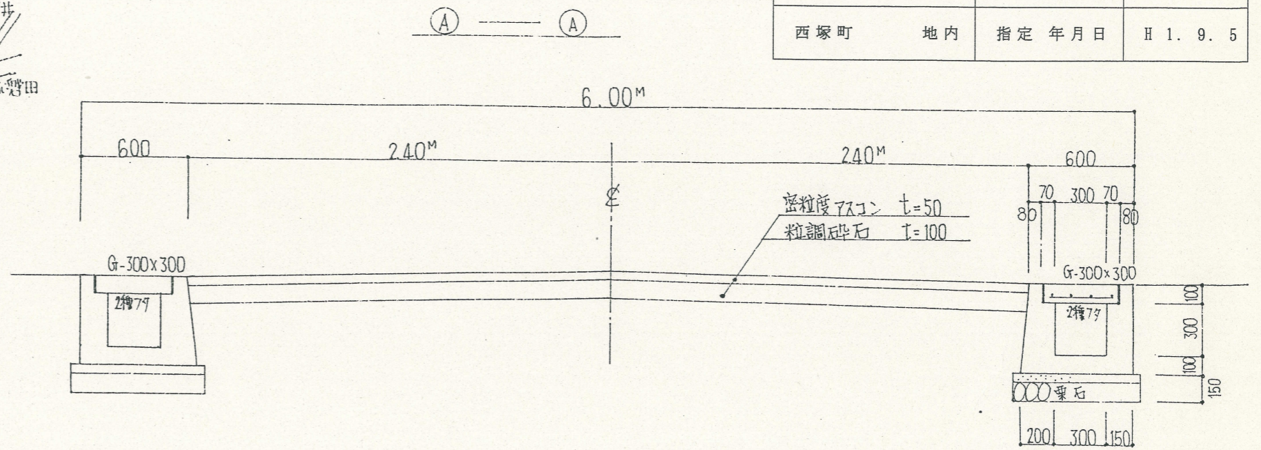
実測図 S = 1:500
