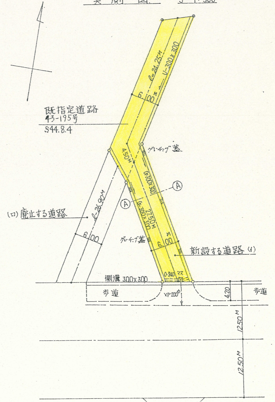
実測図 S = 1:500
