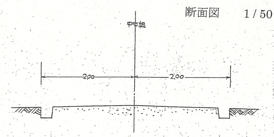
道路断面図 縮尺:1/50
