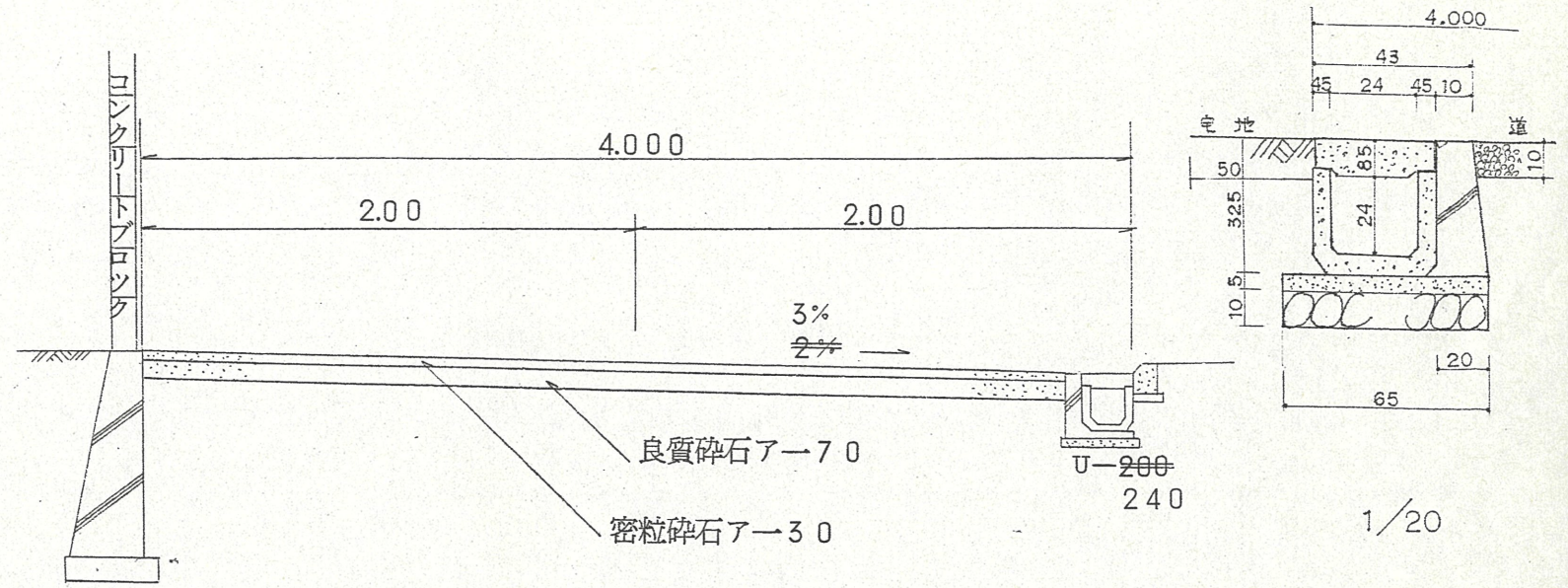
2 断面図 1/30
