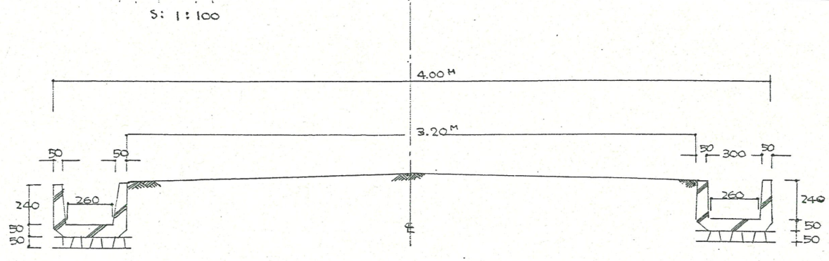
断面図
