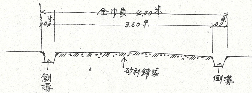
断面図
