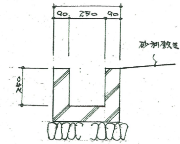
側溝詳細図
