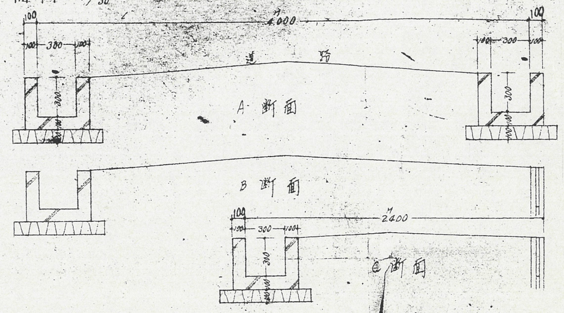
断面図 1/30
