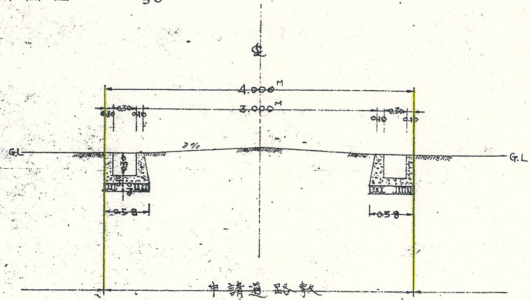
断面図 S = \frac{1}{50}
