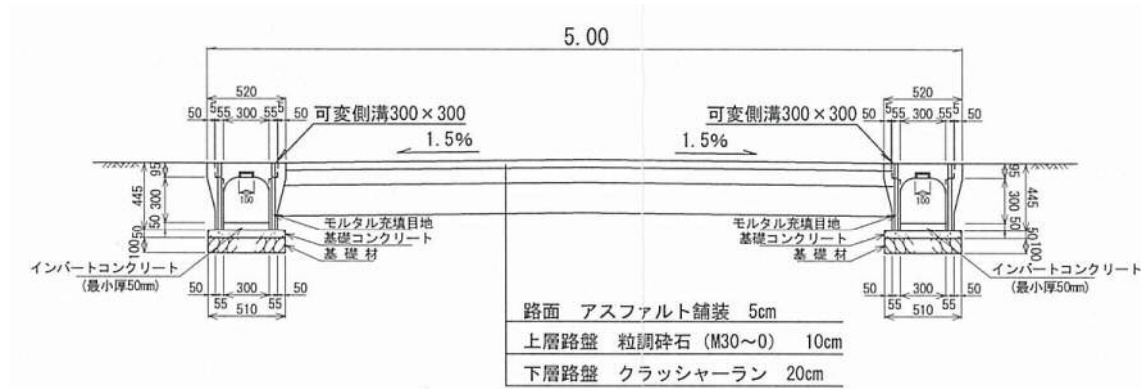
断面図 縮尺: 1/50
