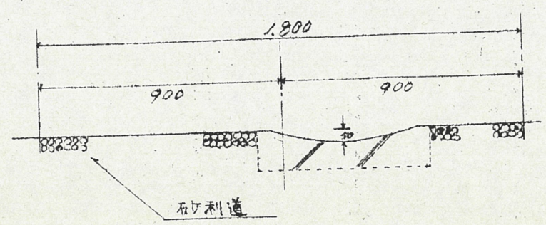
2 断面図 1/20
