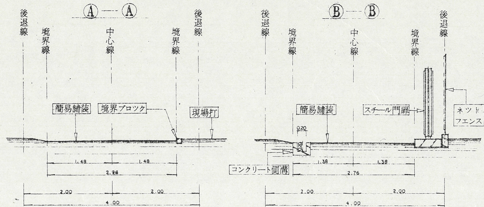
2 断面図
