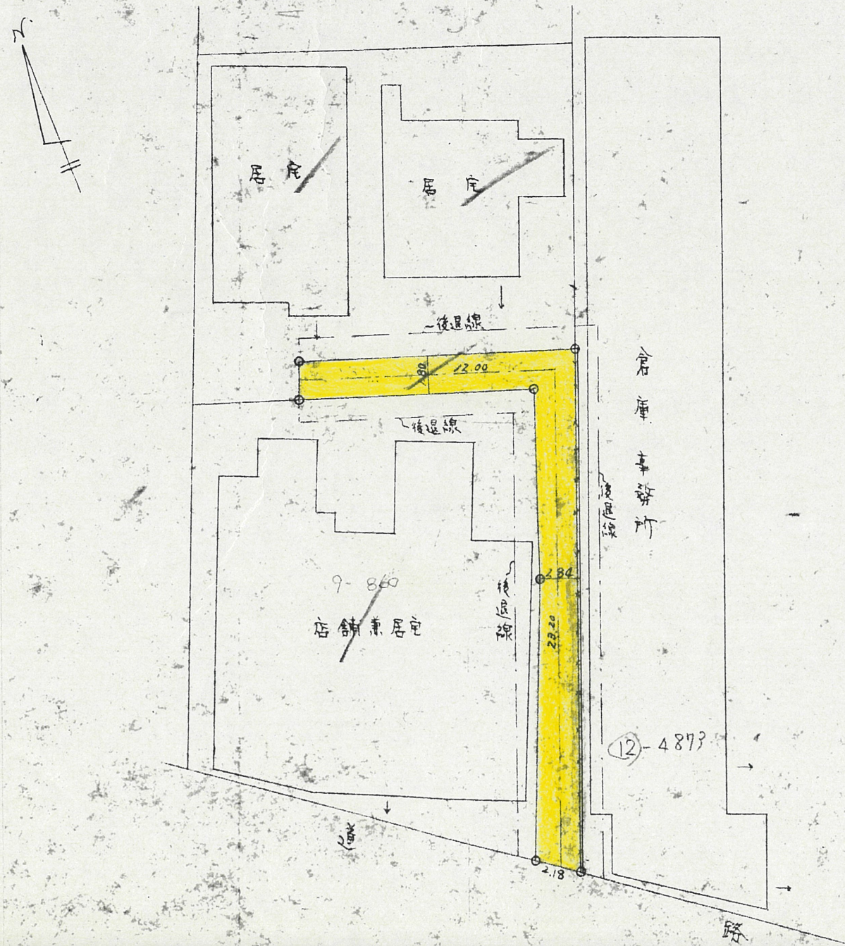
実測図 \frac{1}{250}
