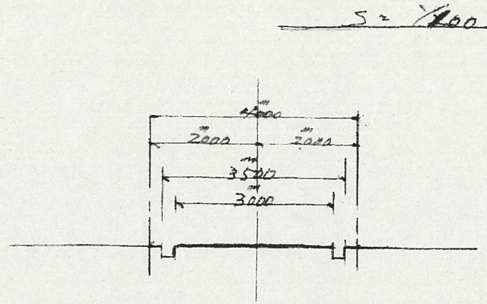
実測断面図
