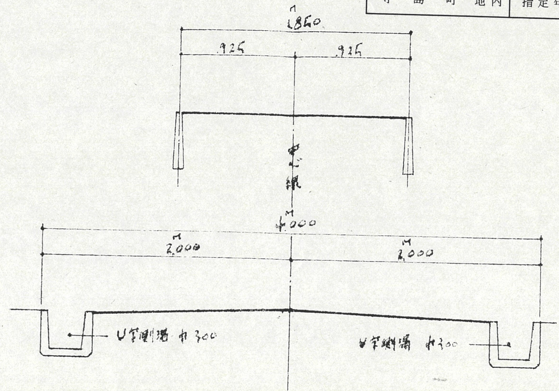
断面図
