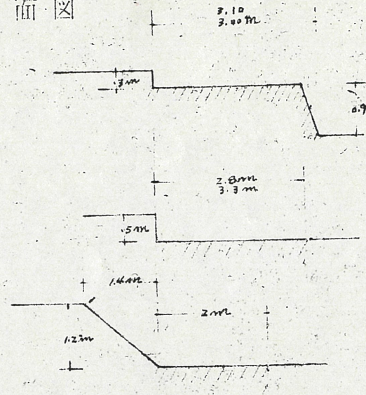
㊦ 平均断面
