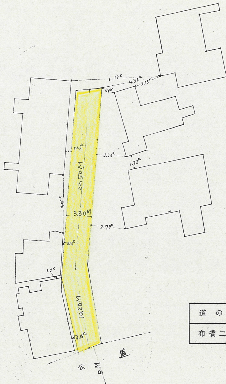
実測図 1/300
