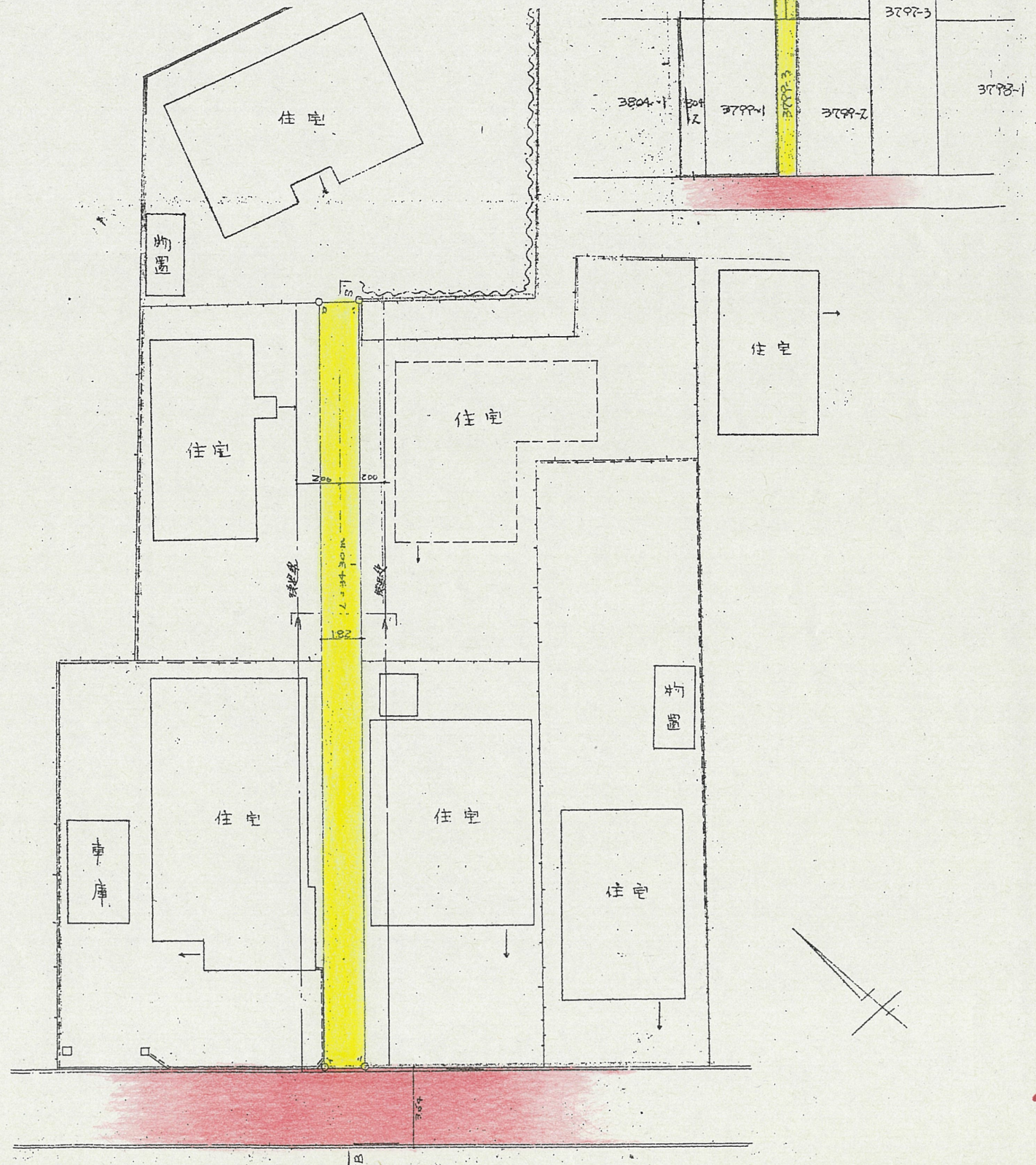
平面図 S=1/250
