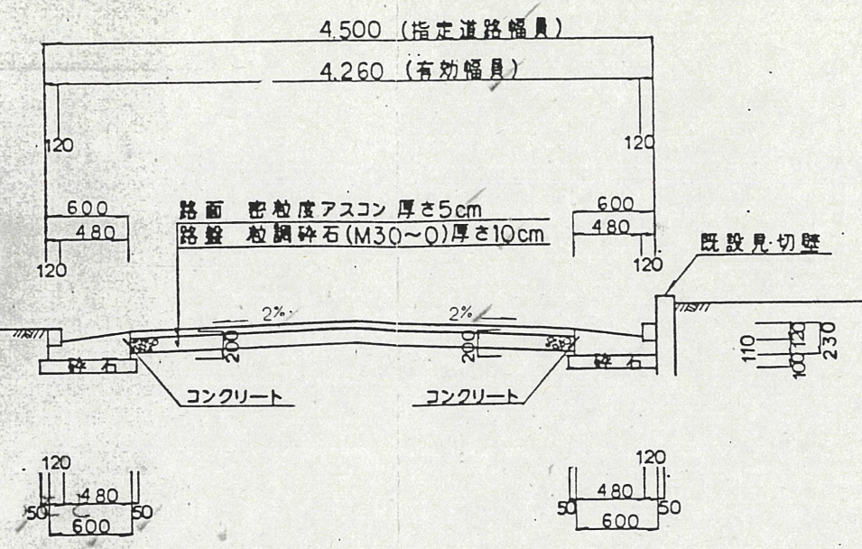
A-A' 断面図 縮尺 1:50
