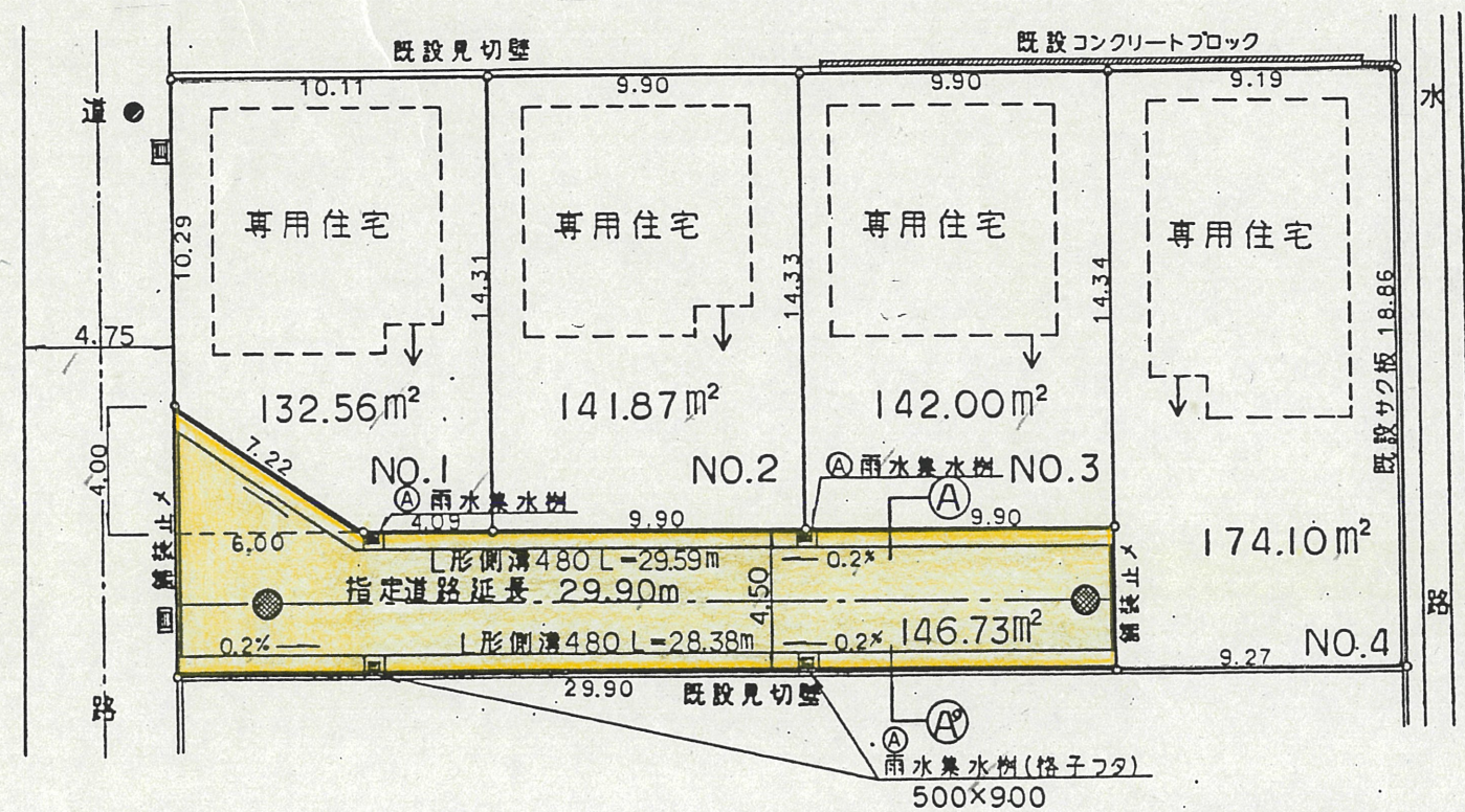
実測図 縮尺 1:250
