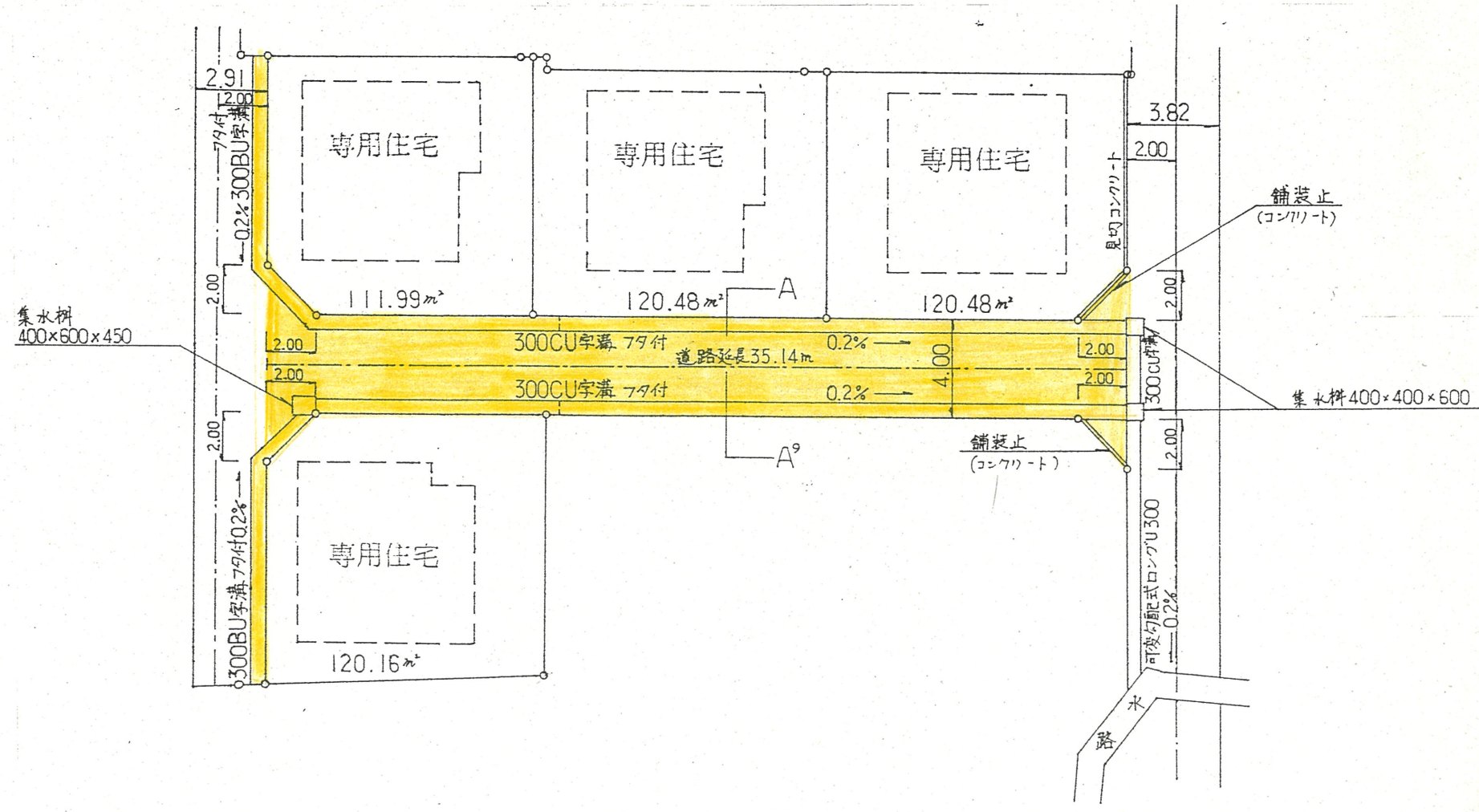
実測図 縮尺 1:250
