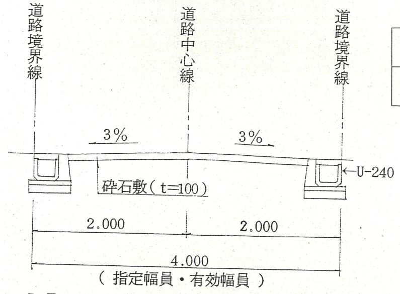
断面図 A ~ A ( S = 1 / 50 )
