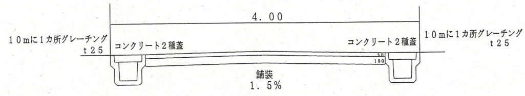
道路断面図
