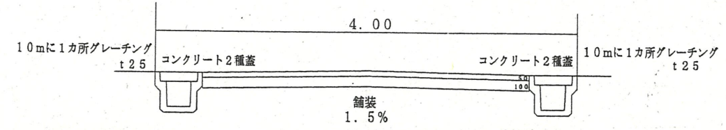
道路断面図
