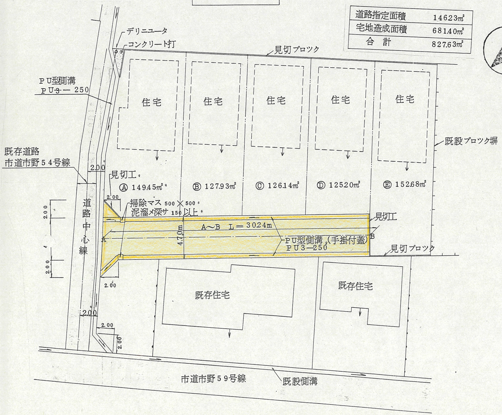
実測図
