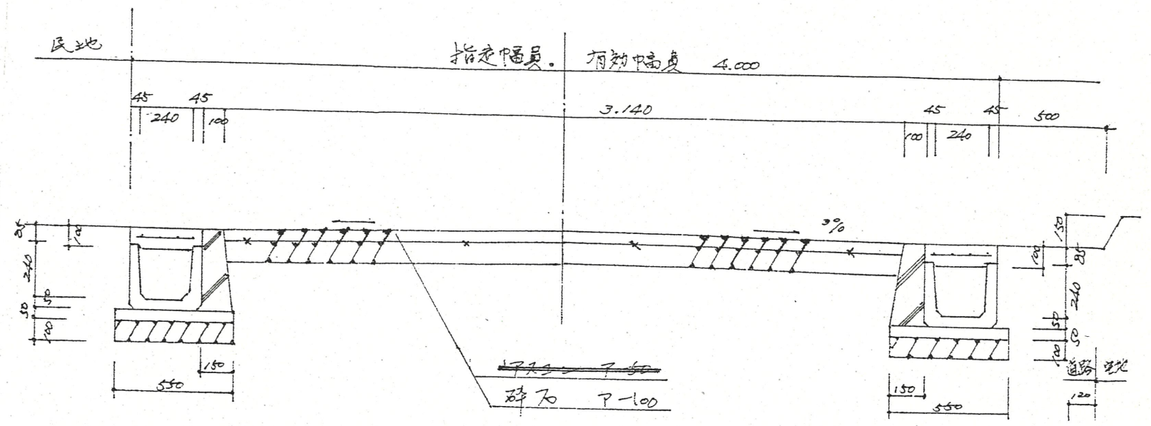
2 断面図 1/25
