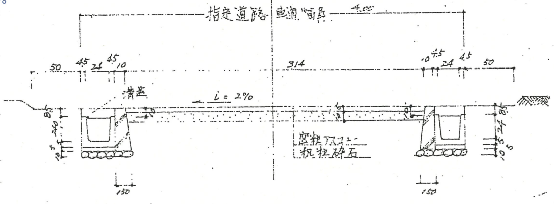
断面図 S = 1 / 40
