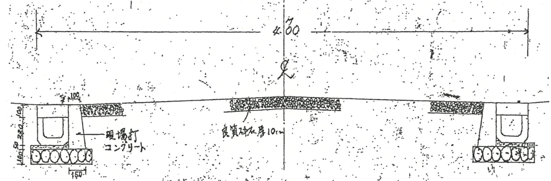
断面図 S=1/30
