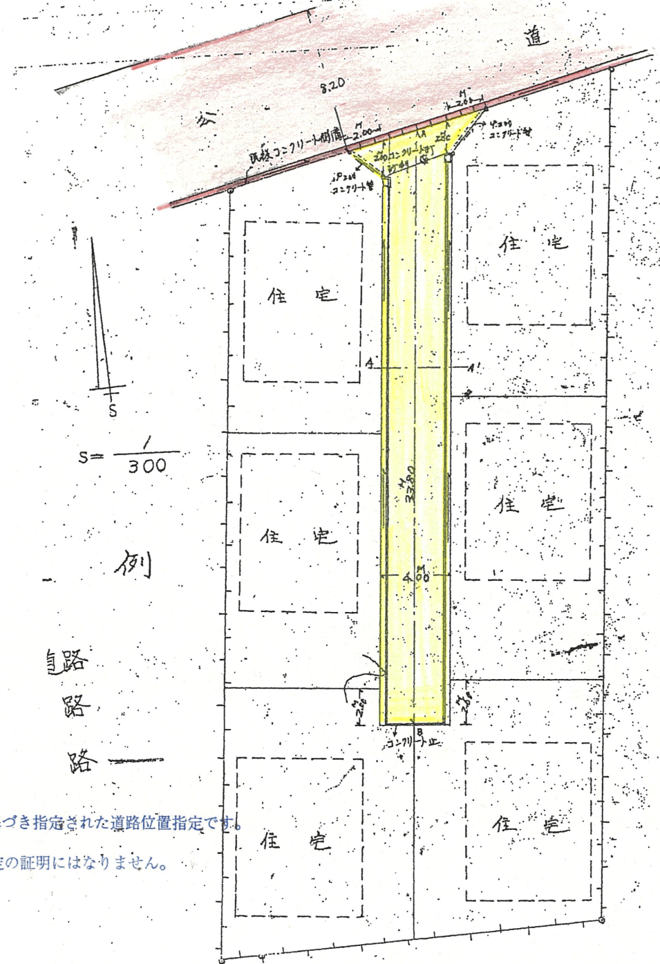
平面図 S=1/300
