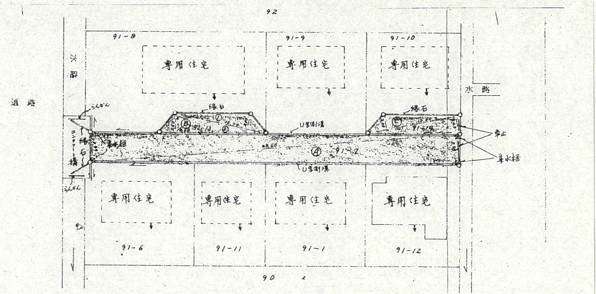
地積測量図 縮尺 1:500
