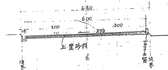
断面図 S = 1 / 100
