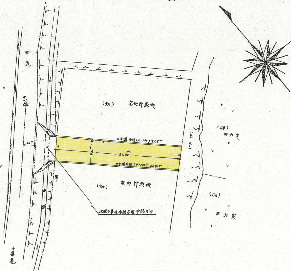
実測 平面図
