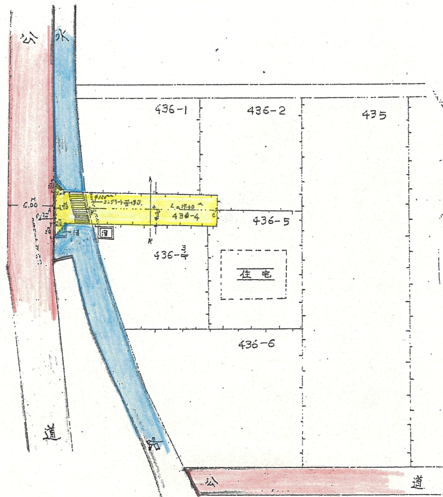
平面図 S = 1 / 500
