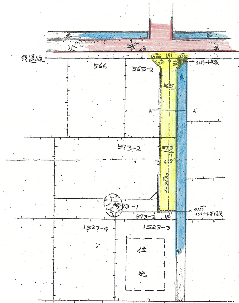
平面図 S = 1 / 500
