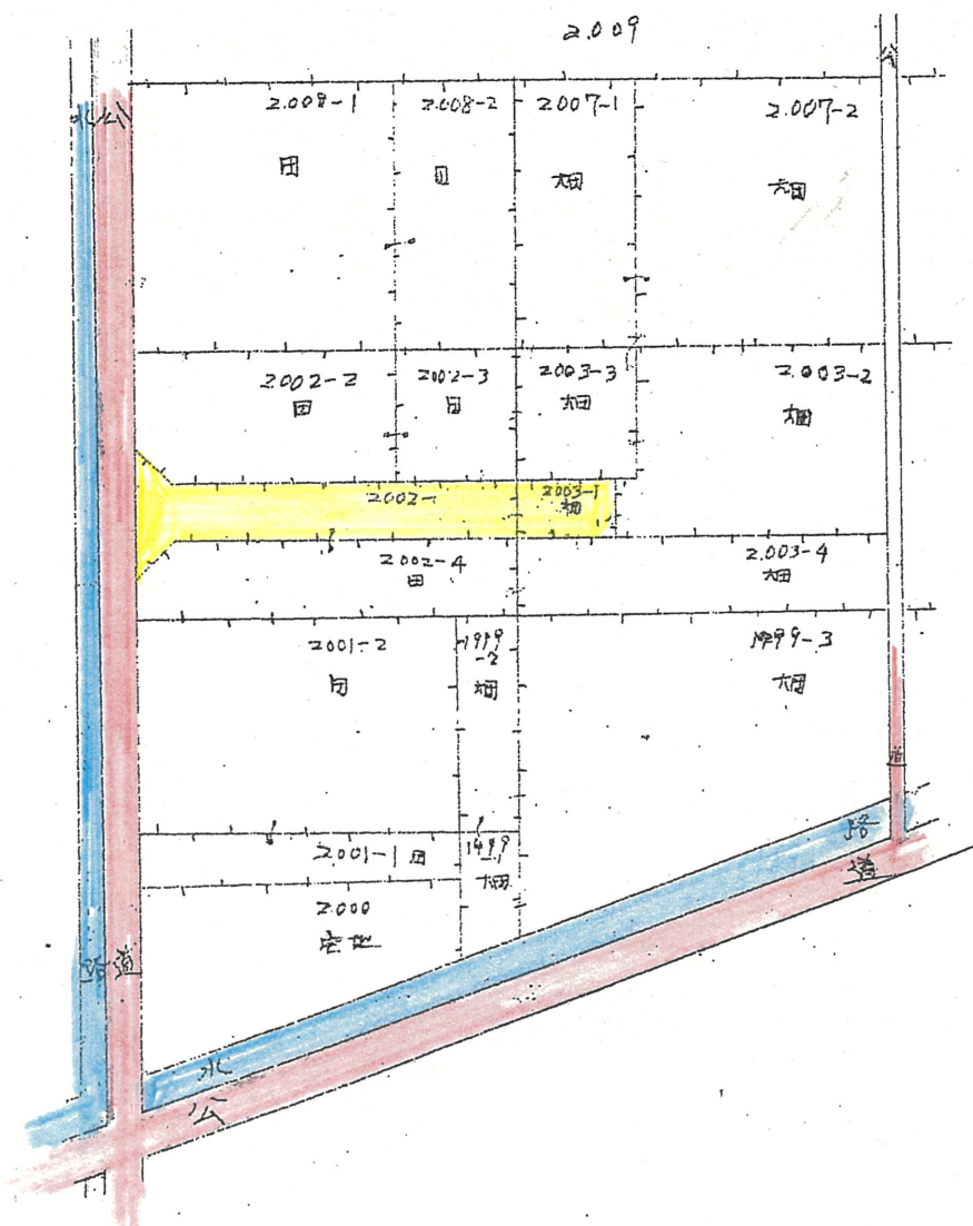
公図写 S = 1 / 600
