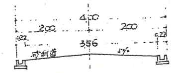
断面図 S = 1 / 100
