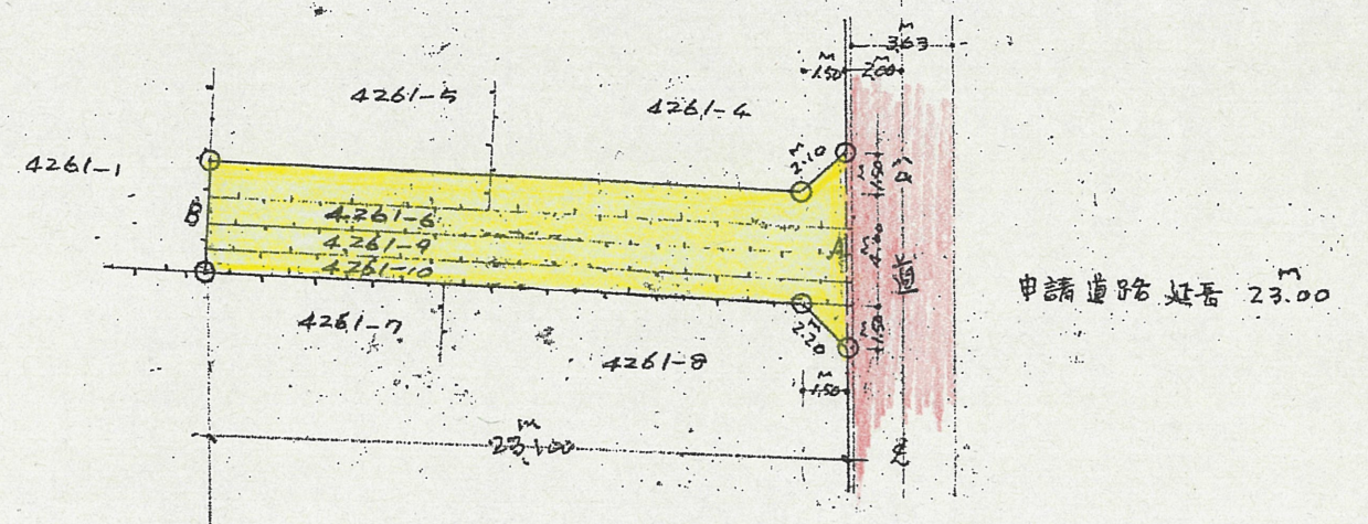
平面図 S = 1 / 300
