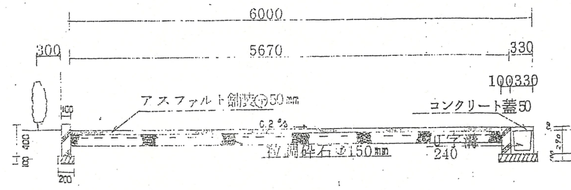
断面図 S = 1 / 50
