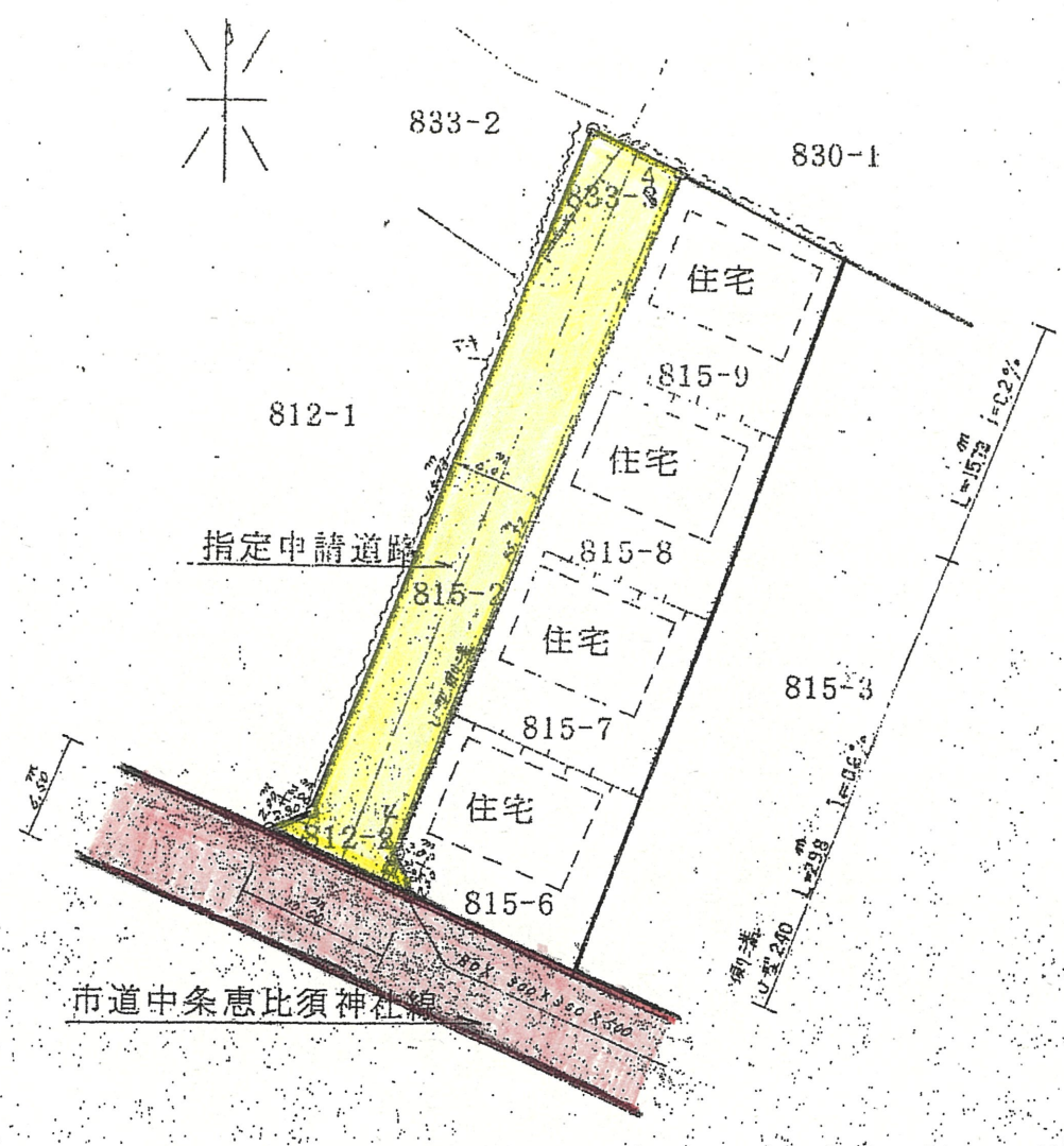
平面図 S = 1 / 500
