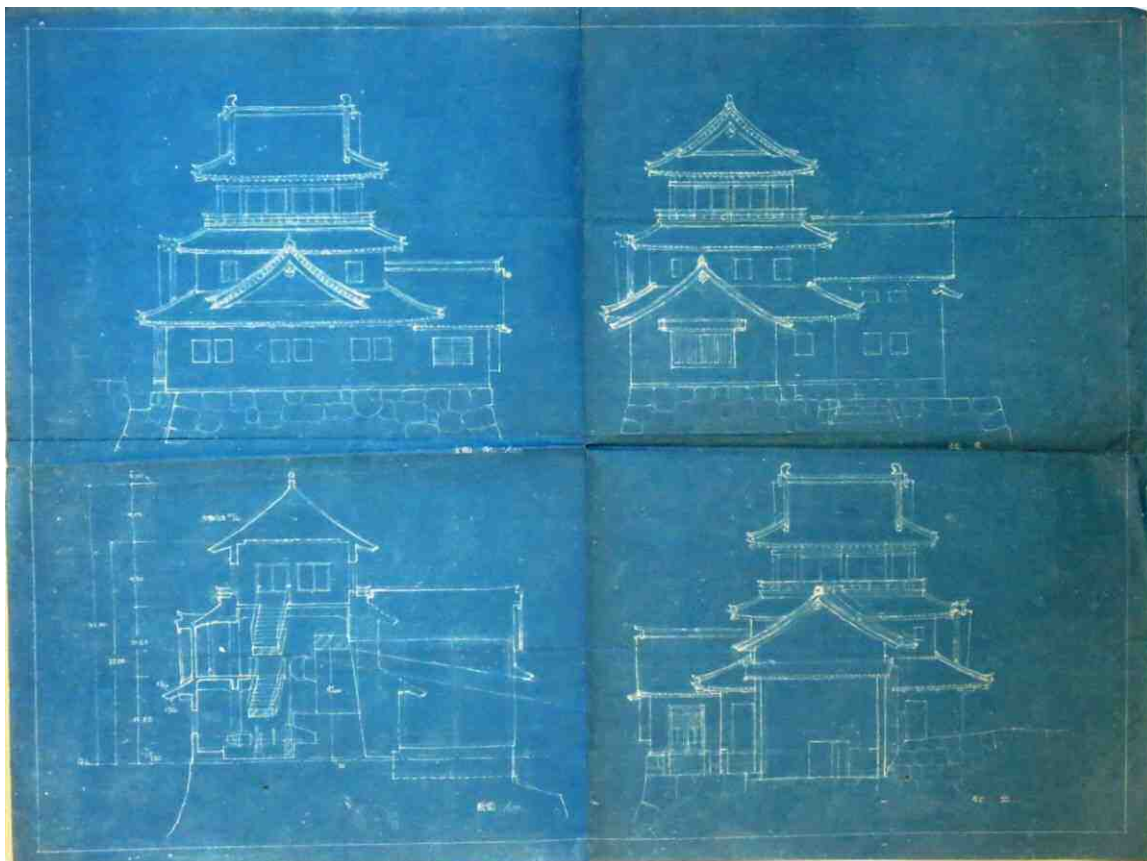
設計図（設計検討案 縦40cm、横52cm）
