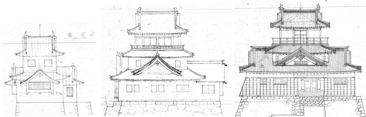
浜松城復興天守閣設計図（左:昭和30年案 中:設計検討案 右:最終案（現況））
