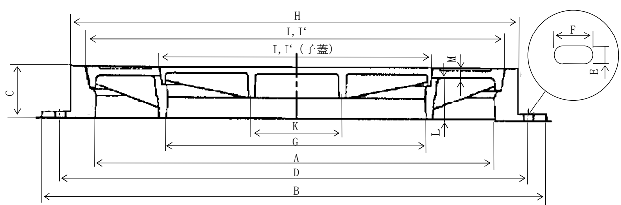
グラウトマンホール呼び 900×600
