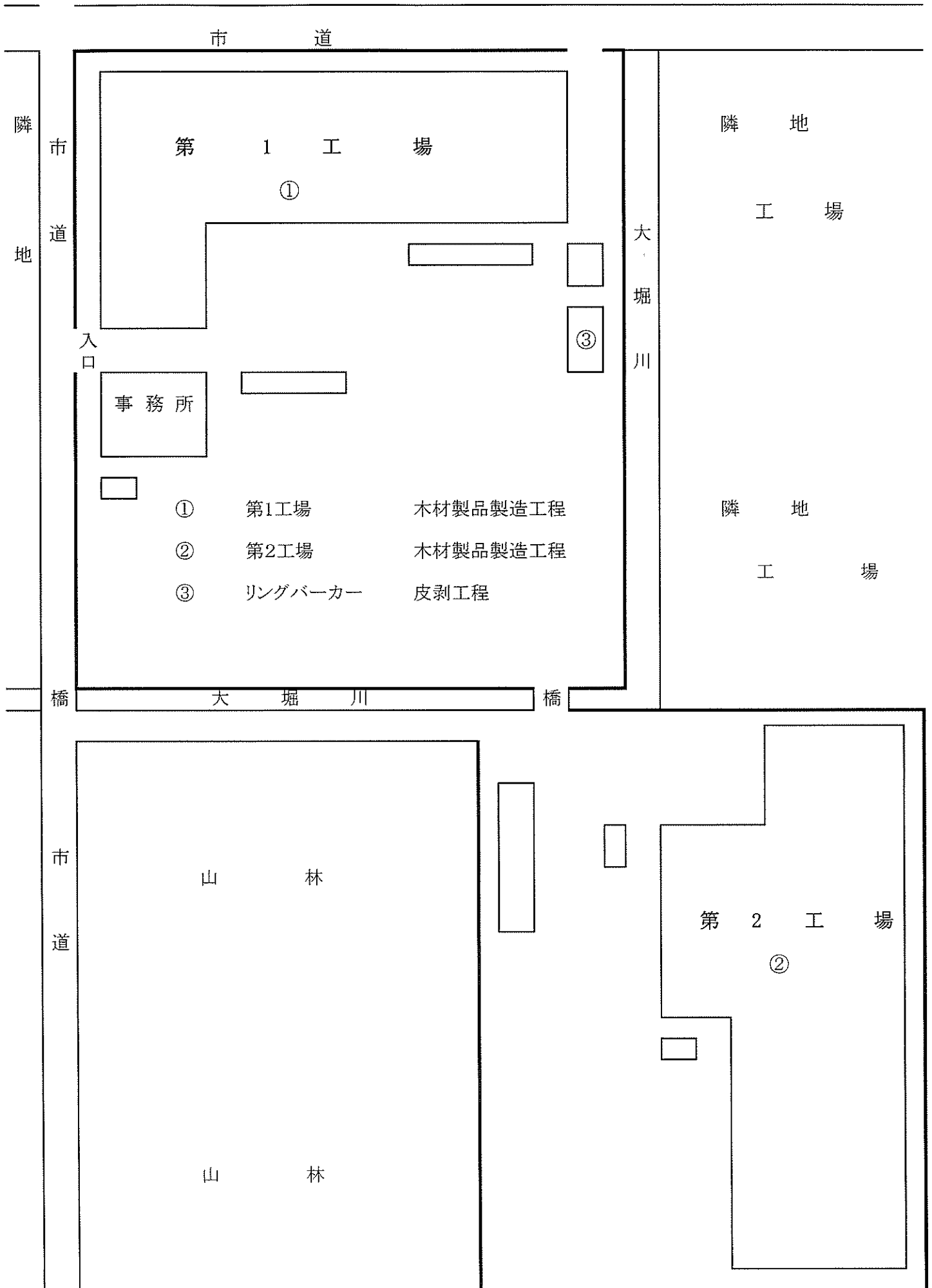
図2 工場配置図 (別紙添付図 図2-A, 図2-B)
