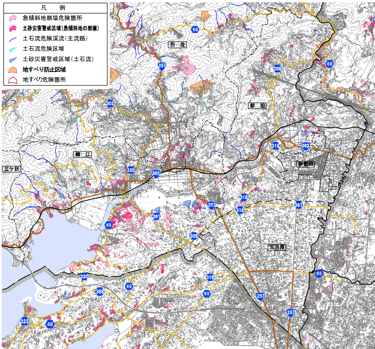
北区における土砂災害危険箇所（細江・三方原・都田・新都田地区）（平成24年3月現在）
