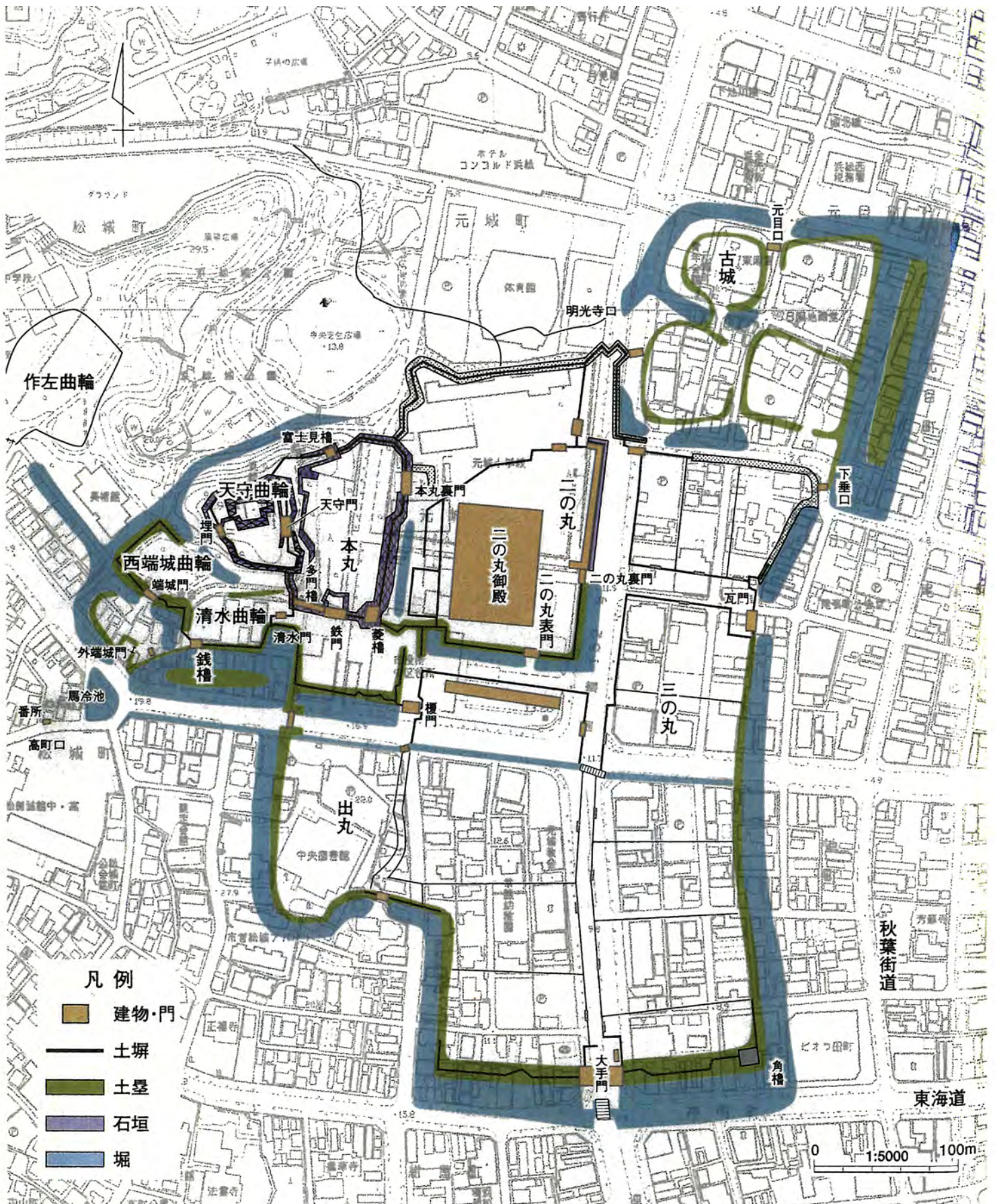
浜松城推定復原図 三の丸をはじめ城域の多くは市街地の中に埋もれている。
