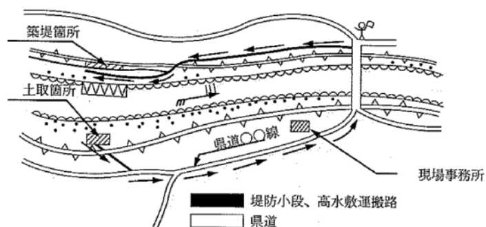
図-1 残土運搬、資材運搬の経路
